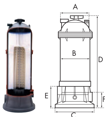
Filtre découpé Star Clear™
